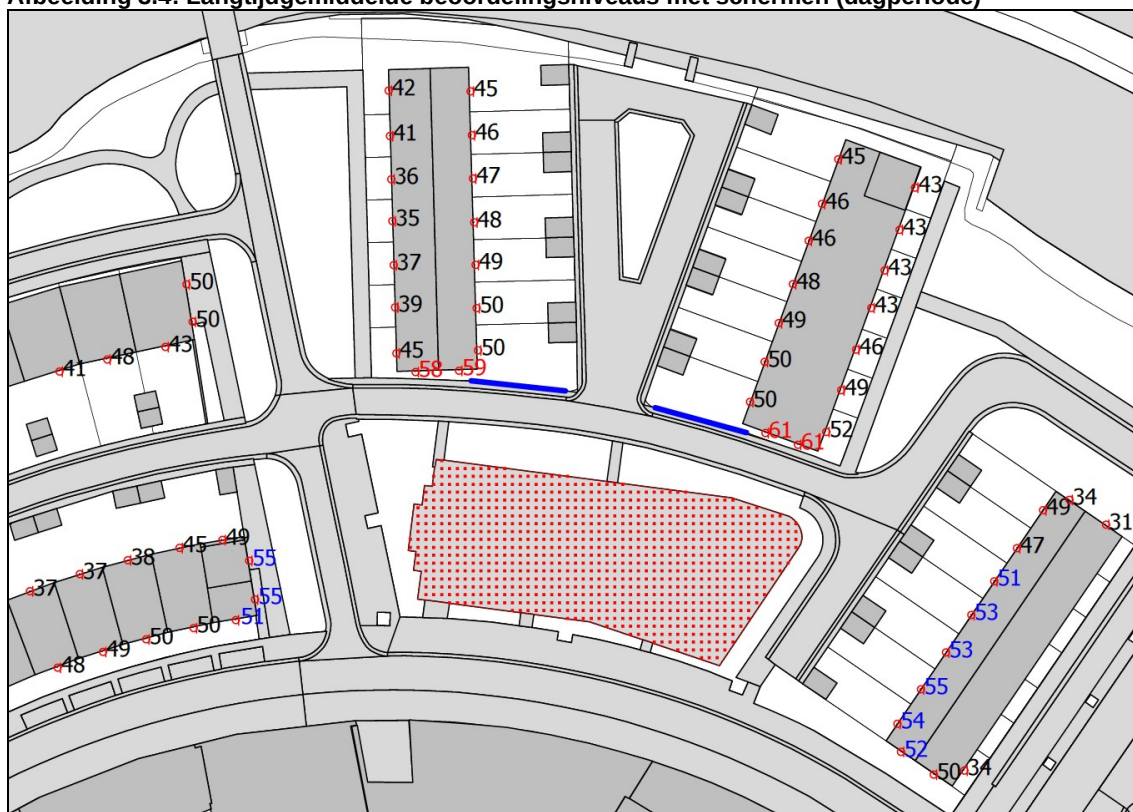
Afbeelding 3.4: Langtijdgemiddelde beoordelingsniveaus met schermen (dagperiode)
