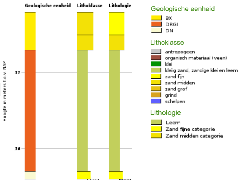
Afbeelding 2.4 Schematische weergave bodemopbouw onderzoekslocatie tot een diepte van 9 m + NAP
