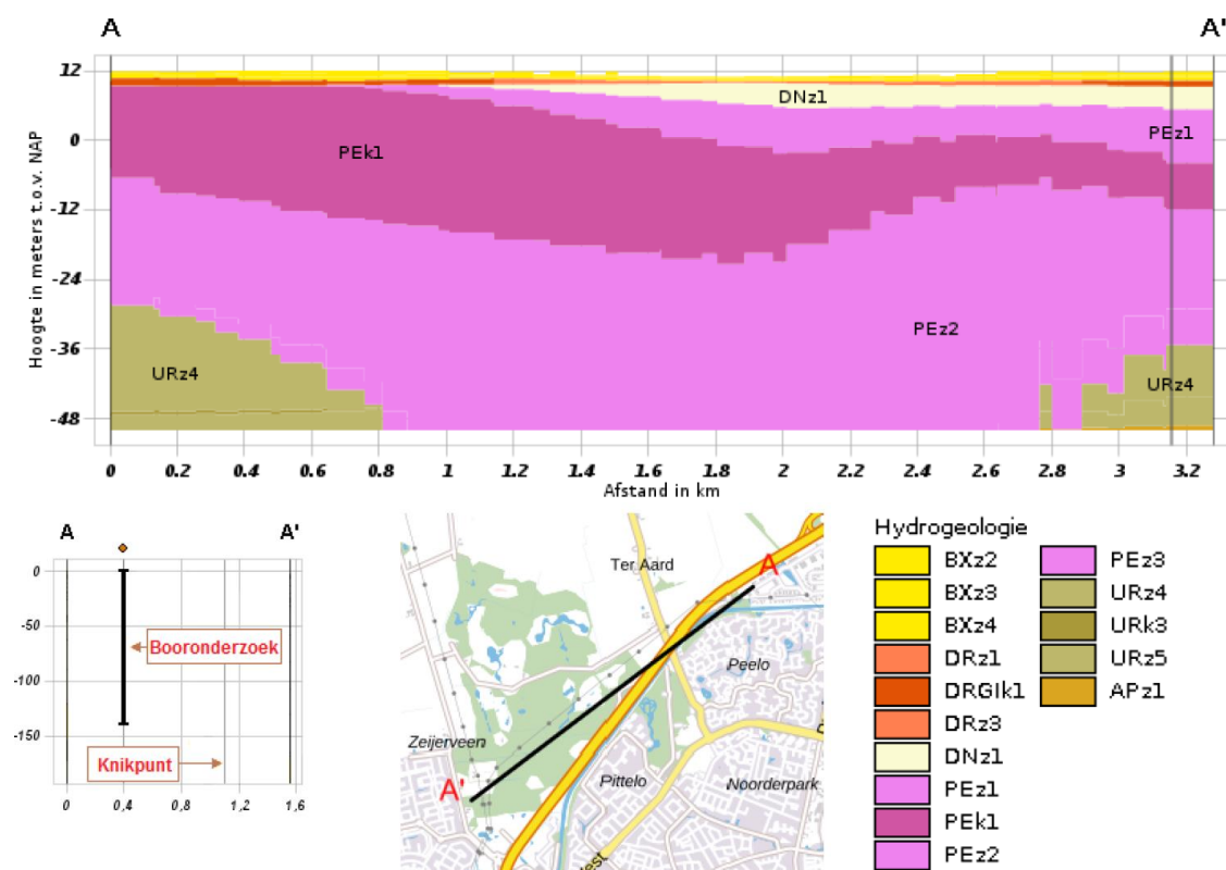
Afbeelding 2.3 Schematische bodemopbouw onderzoekslocatie
