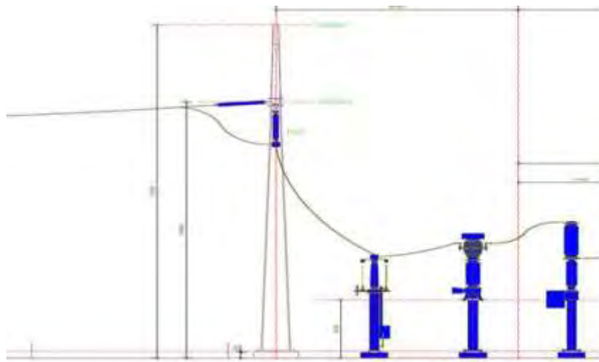
Figuur 4.7 Illustratie dwarsdoorsnede componenten transformatorveld en aansluiting op portaal (nieuwe componenten in blauw)
