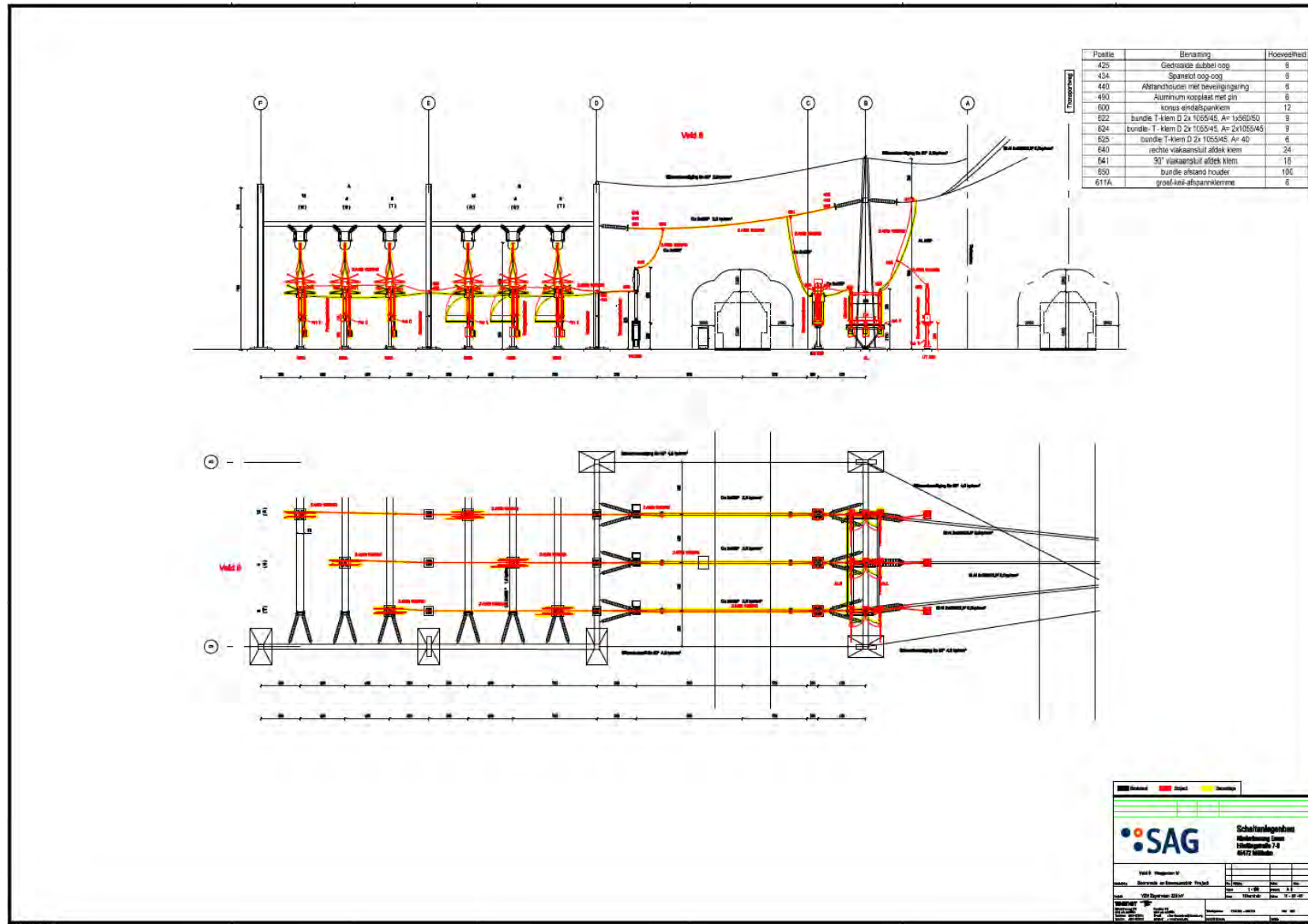
Bijlage C-5 Tekening zijaanzicht 220kV lijnveld 7 en 8
