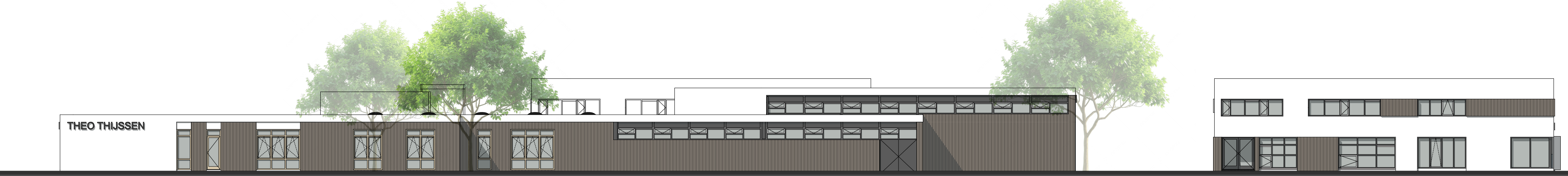
NOORDOOSTGEVEL SCHOOL EN GYMZAAL
