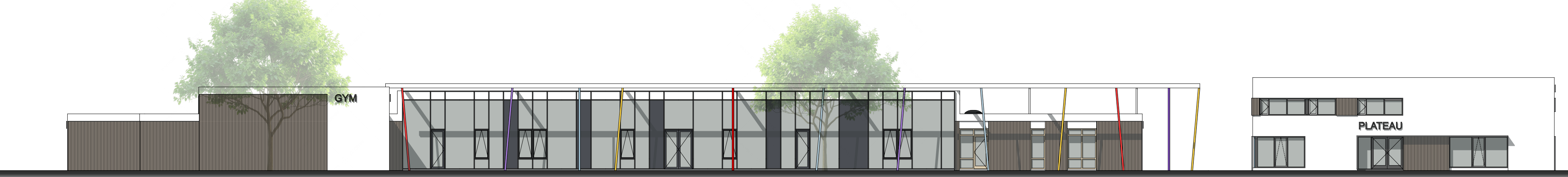
NOORDWESTGEVEL SCHOOL EN GYMZAAL
